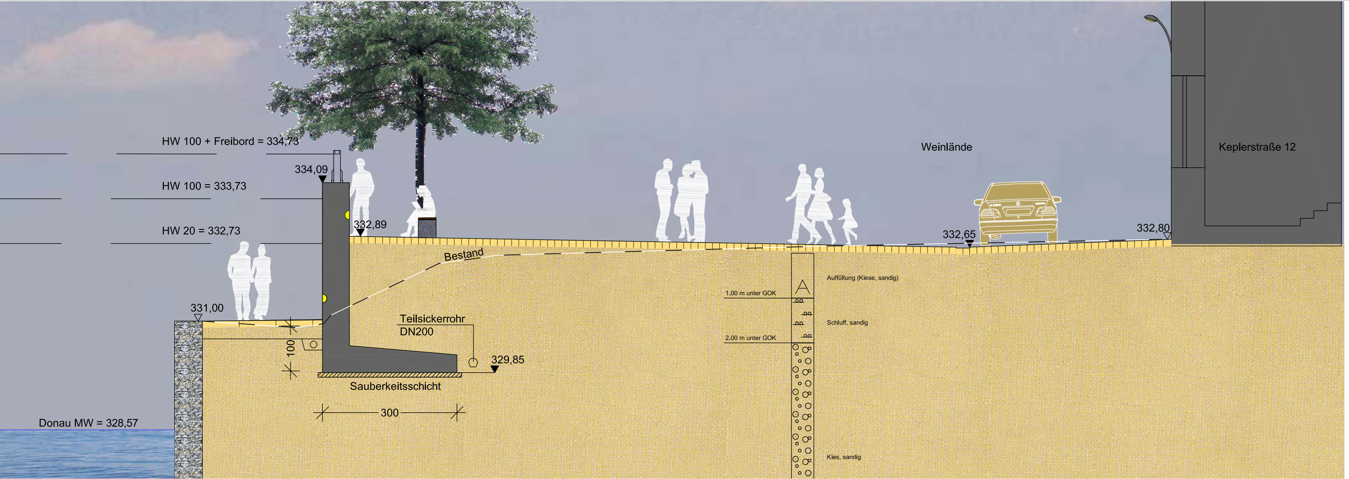
SCHNITT M 1:50
