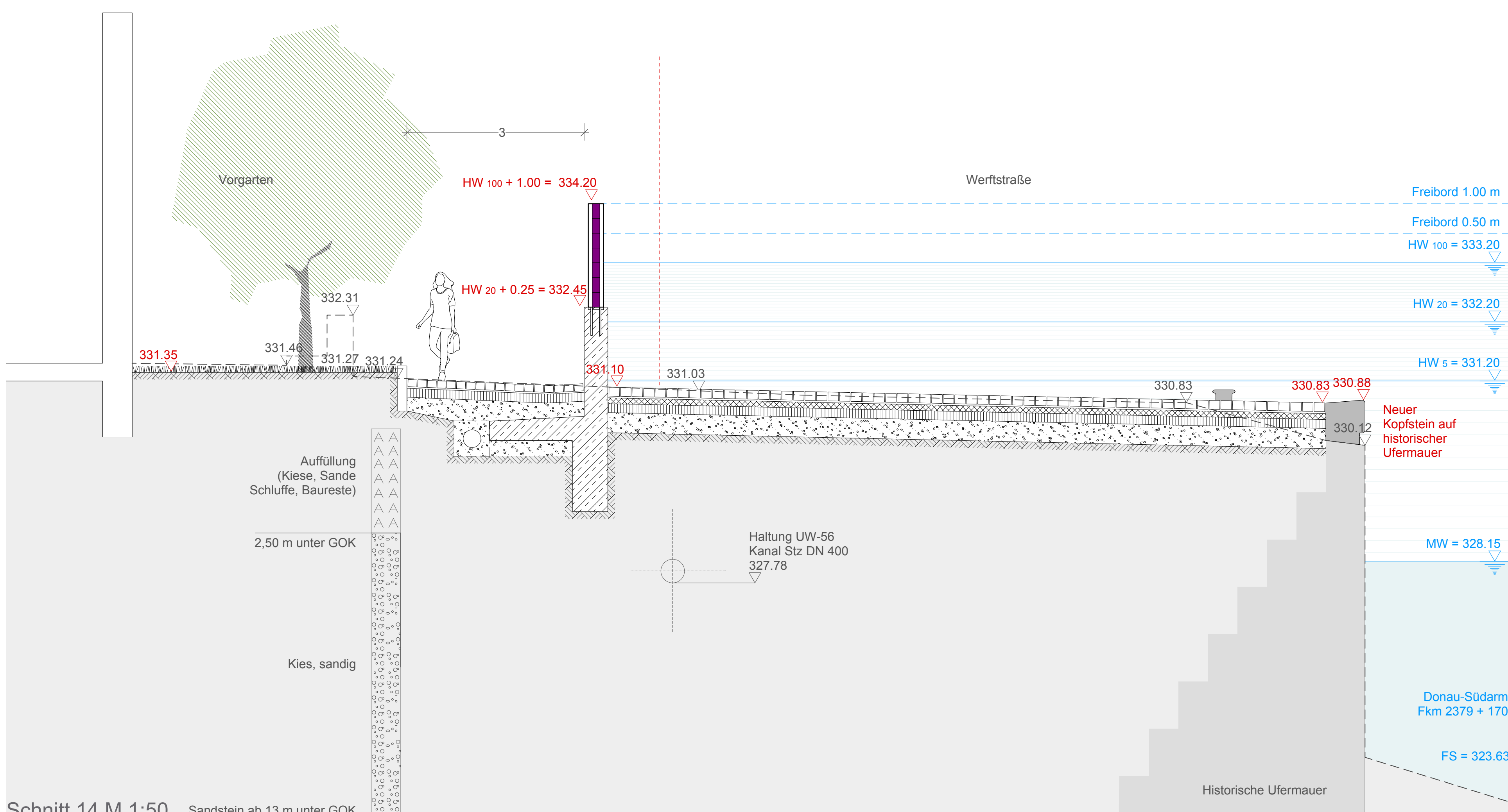
Schnitt 14 M 1:50 Sandstein ab 13 m unter GOK
